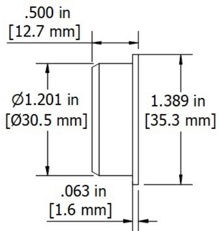
GROMMET
