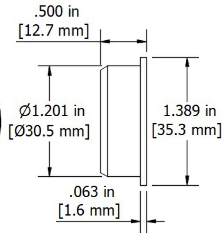
GROMMET
